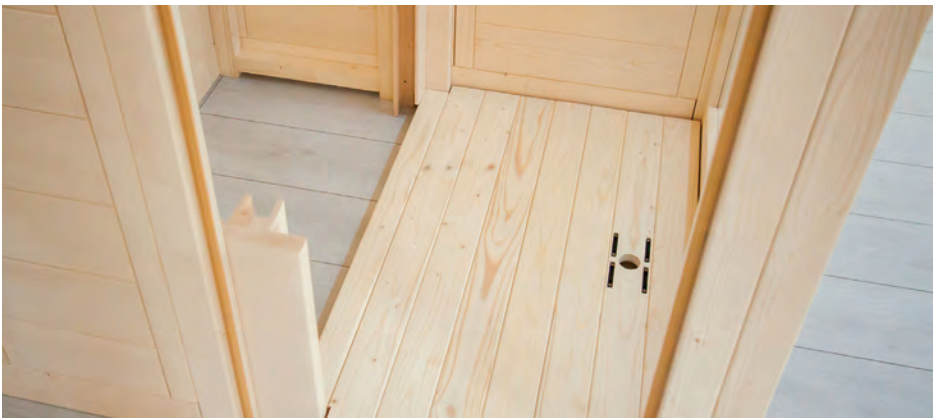
Abb. 19: Fußboden einlegen
